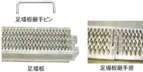
足場板
